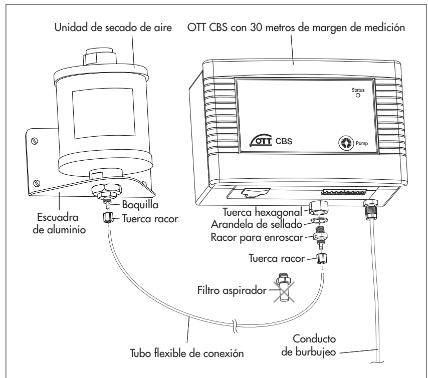
Fig. 1: Esquema de conexión de la unidad de secado de aire al OTT CBS.
