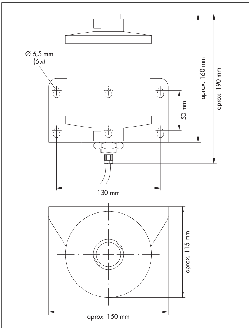
Fig. 3: Medidas de la unidad de secado de aire OTT CBS.
