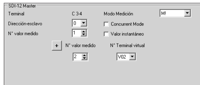
Fig. A2: Ajuste los parámetros de operación del bloque funcional SDI-12 Master del OTT netDL.
