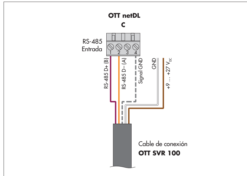
Fig A1: Conexión del OTT SVR 100 con la interfaz RS-485 (protocolo SDI-12 al OTT netDL.
