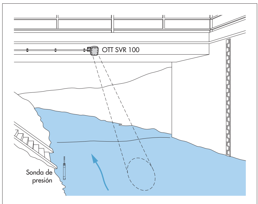
Fig. 3: Ejemplo de aplicación 1: Montaje del OTT SVR 100 en un puente.
