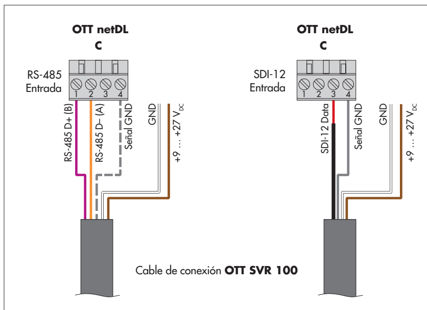
Fig A1: Conexión del OTT SVR 100 con la interfaz RS-485 (protocolo SDI-12; a la izquierda) o con la interfaz SDI-12 (a la derecha) al OTT netDL.
