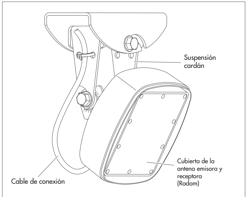
Fig. 2: Sensor de radar OTT SVR.
