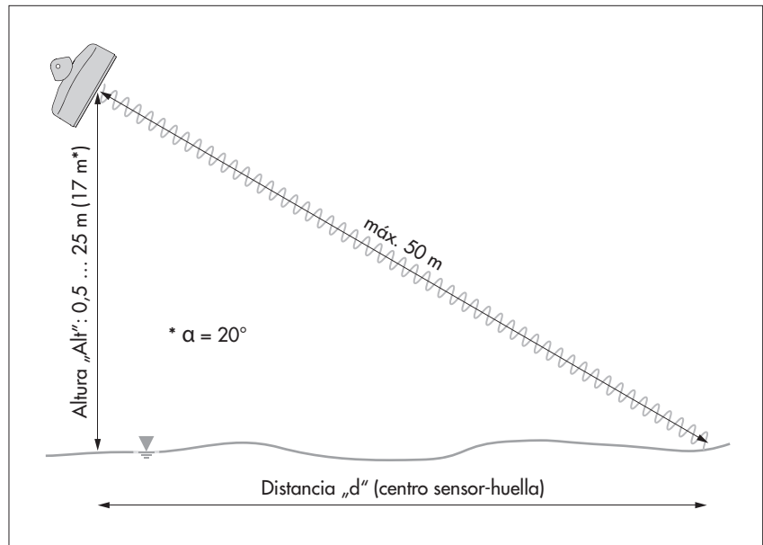
Fig. 7: Distancia máxima del OTT SVR 100 respecto a la superficie del agua.
