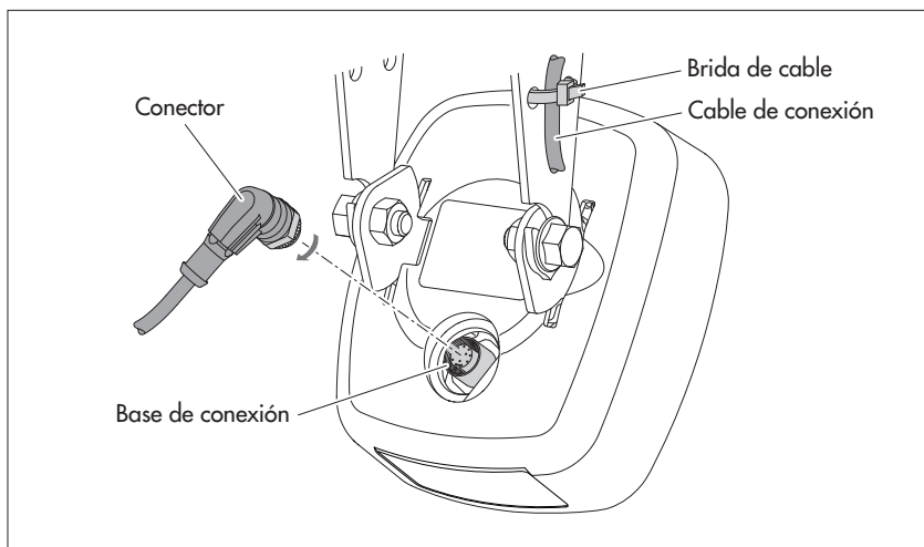
Fig. 9: : Conexión del conector angular del cable al OTT SVR 100.
