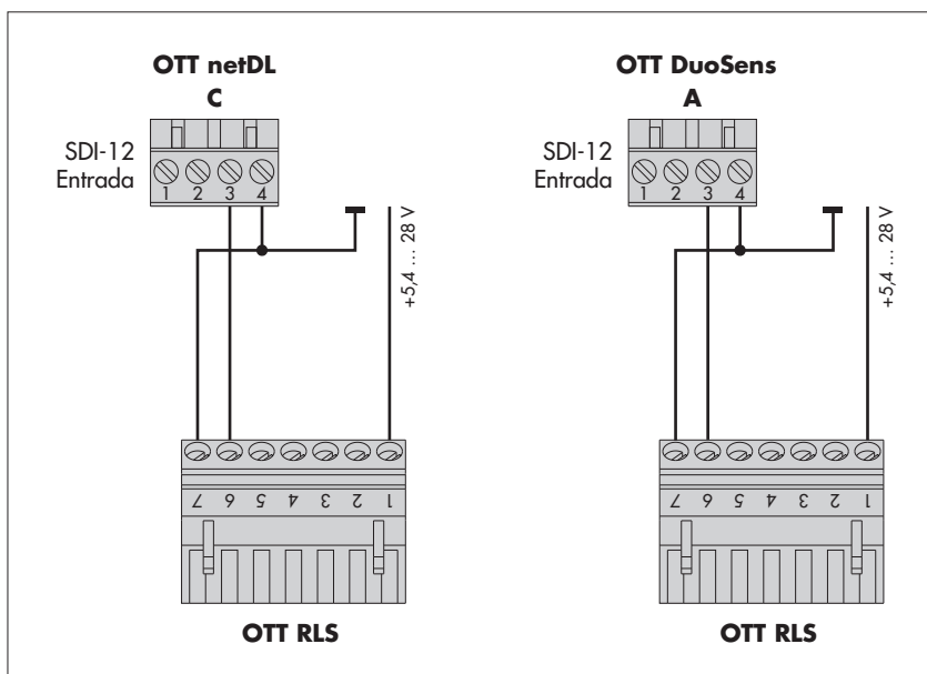
Fig. 10: Conexión de OTT RLS a OTT netDL o OTT DuoSens mediante la interfaz SDI-12. Las letras sobre los elementos atornillados de emborne identifican las conexiones posibles a OTT netDL/OTT DuoSens.
