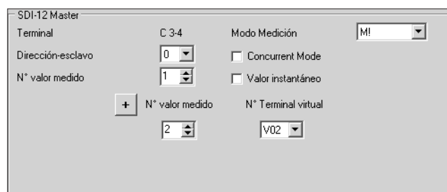
Fig. 12: Configuración de los parámetros de servicio del bloque funcional SDI-12 Master de OTT netDL o DuoSens.
