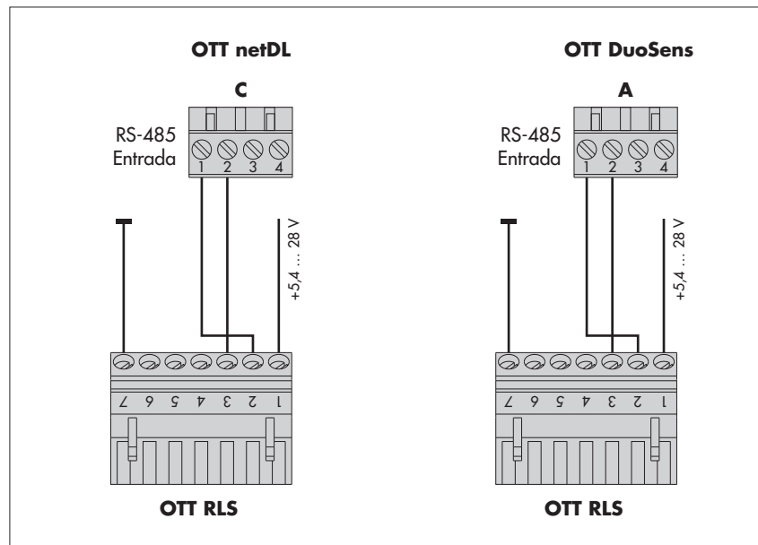
Fig. 11: Conexión de OTT RLS a OTT netDL o a OTT DuoSens mediante la interfaz RS-485 (protocolo SDI-12).
