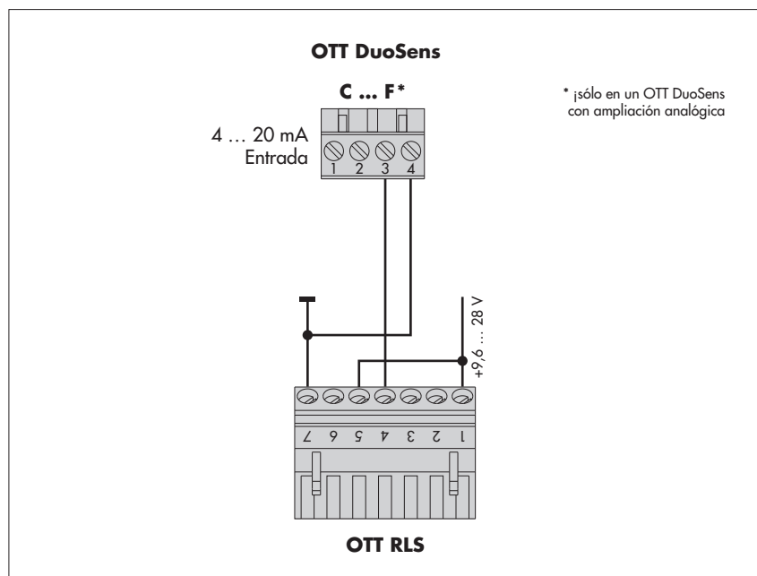
Fig. 14: Conexión del OTT RLS a OTT DuoSens mediante la interfaz 4 ... 20 mA.
