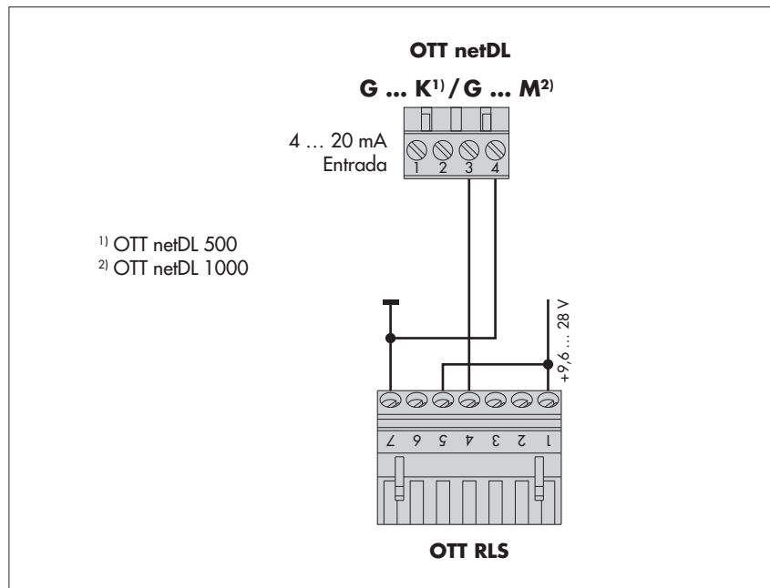
Fig. 13: Conexión del OTT RLS a OTT netDL mediante la interfaz 4 ... 20 mA.
