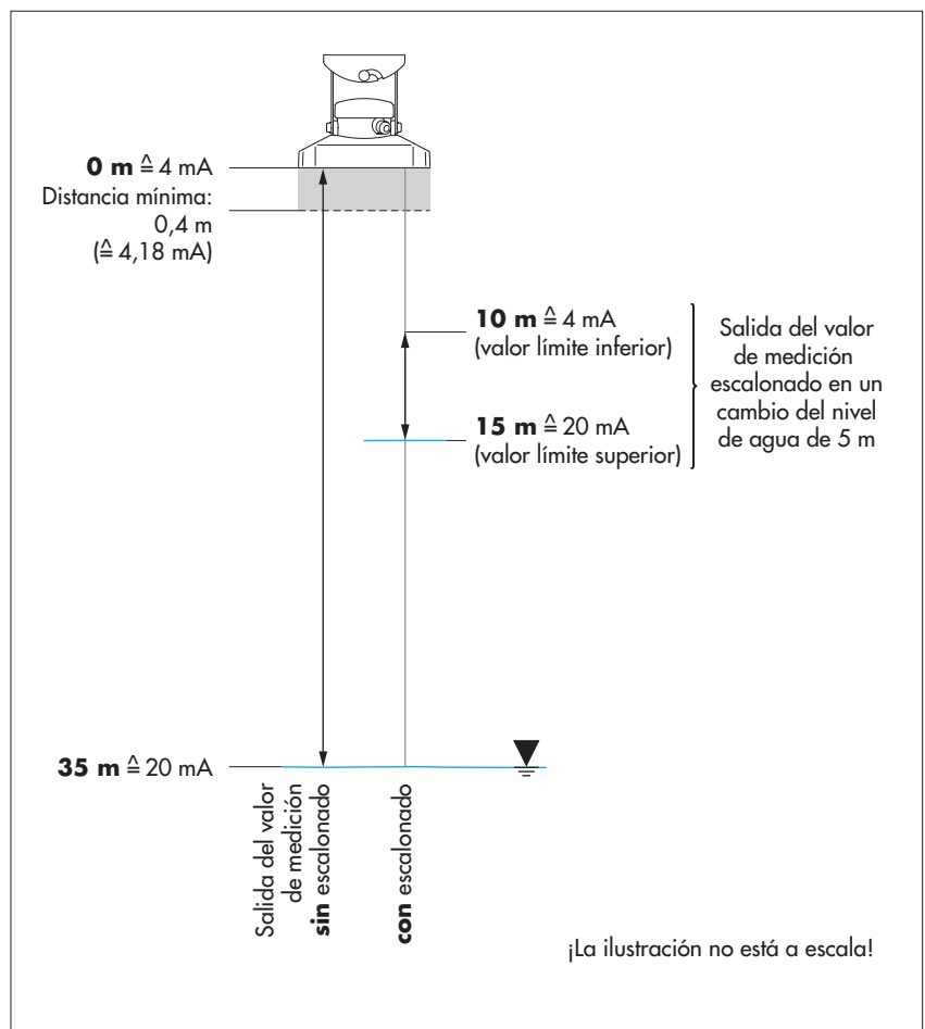
Fig. 9: Escalonado de la salida del valor de medición de la interfaz 4 ... 20 mA a un margen de medición menor.
