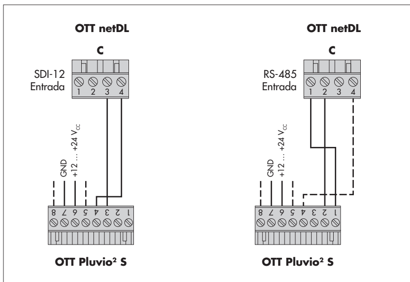
Fig. A1: Conexión del OTT Pluvio 2 S al OTT netDL mediante la interfaz SDI-12.
