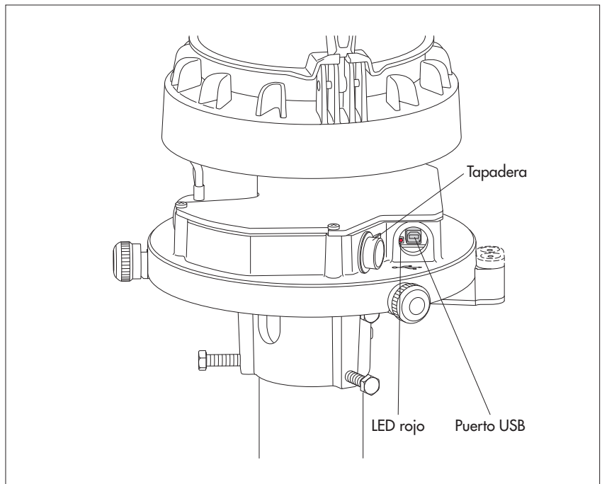
Fig. 18: Realización del control de funcionamiento.
