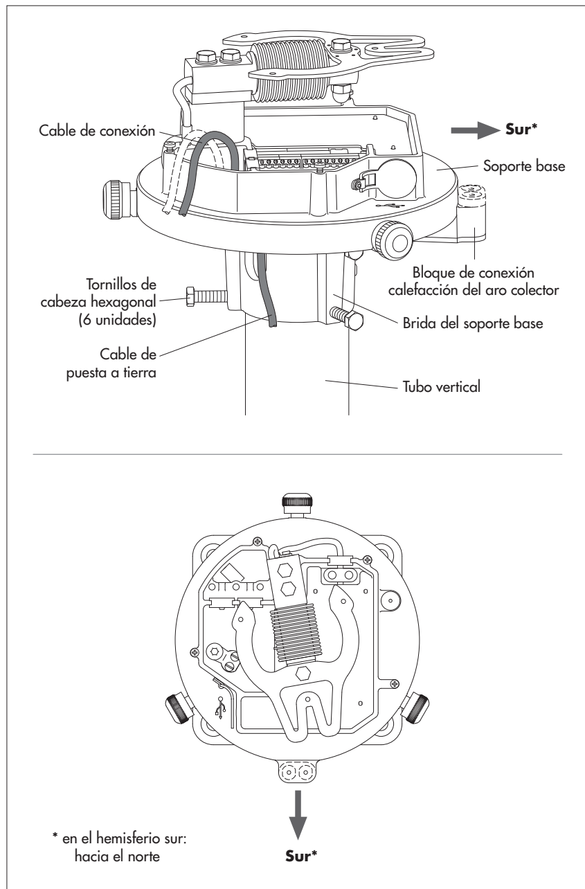
Fig. 12: Instalación del soporte base sobre el tubo vertical.
