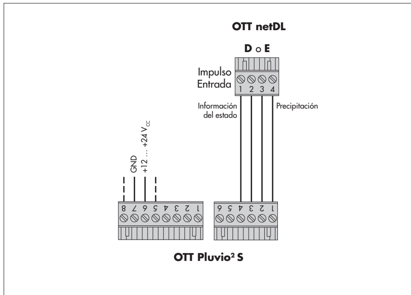
Fig. A4: Conexión del OTT Pluvio 2 S al OTT netDL mediante la salida de impulsos.
