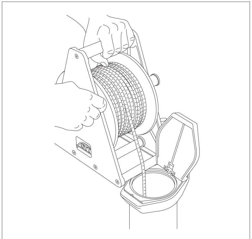
Abb. 3: Anwendungsbeispiel Abstichmessung mit dem Kabellichtlot KL 010 TCM.
