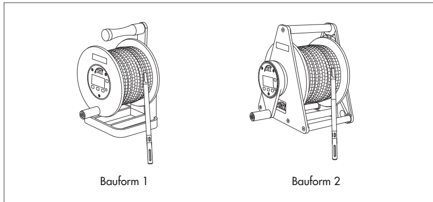
Abb. 1: Das Kabellichtlot KL 010 TCM gibt es in zwei Bauformen: Bauform 1 bis 100 m Messbandlänge; Bauform 2 ab 150 m Messbandlänge.
