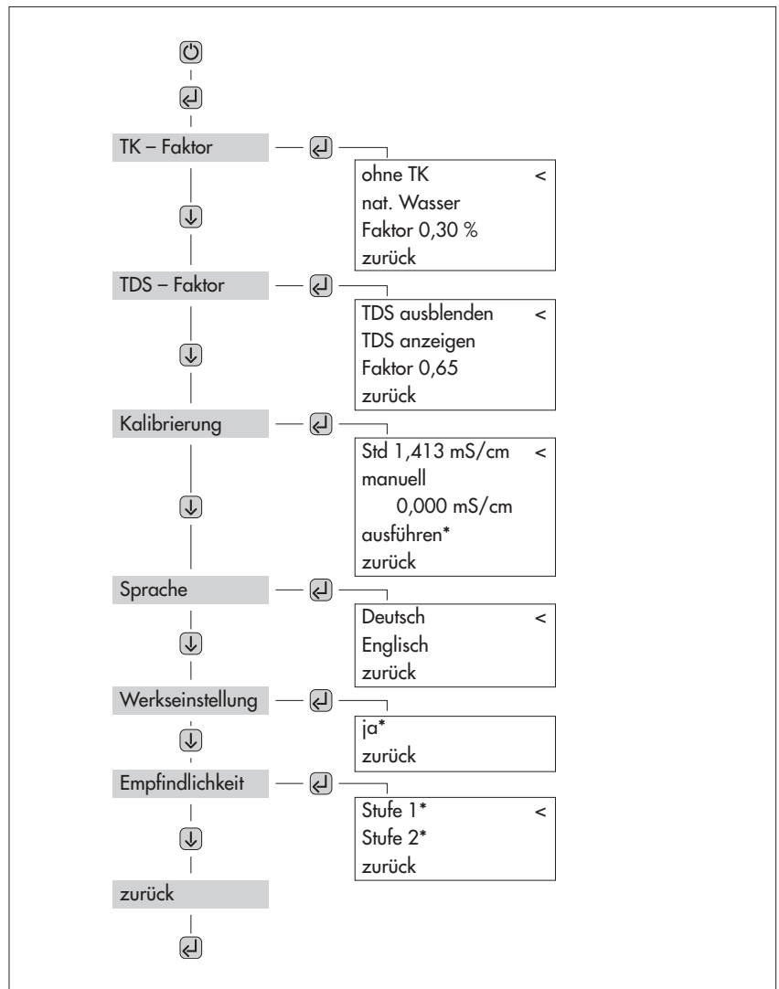
Abb. 2: Struktur des Grundeinstellungs-Menüs.
