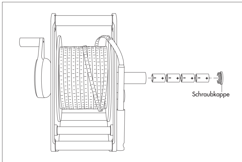
Abb. 4: Batterien wechseln (Bauform 2).
